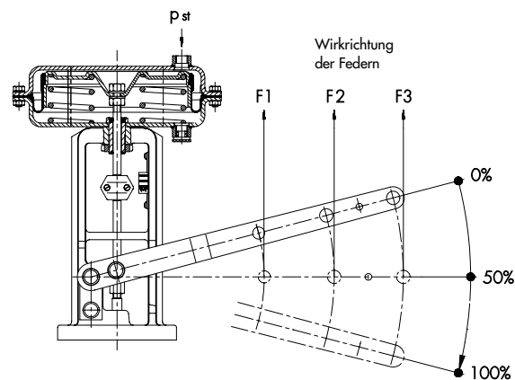
Bild 6 · Wirkbild, Ausführung "Antriebsstange einfahrend" Hebelstellung bei p_{st} = 0 bar (Stellweg 0 %)
