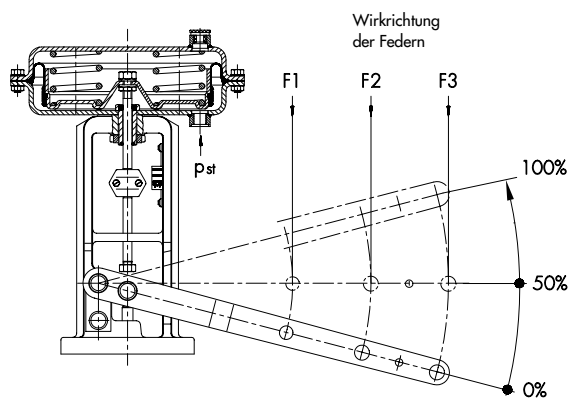
Bild 5 · Wirkbild, Ausführung "Antriebsstange ausfahrend" Hebelstellung bei p_{st} = 0 bar (Stellweg 0 %)
