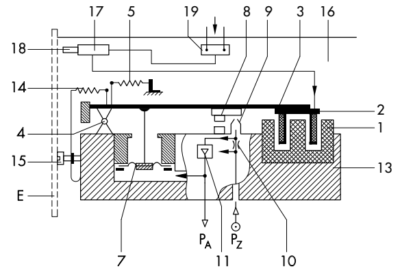
Bild 8 · Wirkbild des i/p-Stellumformers (Einschubgerät)
