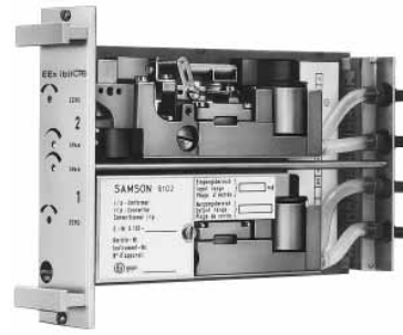
Bild 5 · 2fach-i/p-Stellumformer Typ 6102-72 mit eigenem Eingangsstromkreis EEx ib II C
