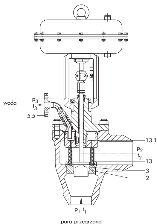
Rys. 4 · Zawór schładzający do pary typu 3286-1 z końcówkami do wspawania i siłownikiem typu 3271
