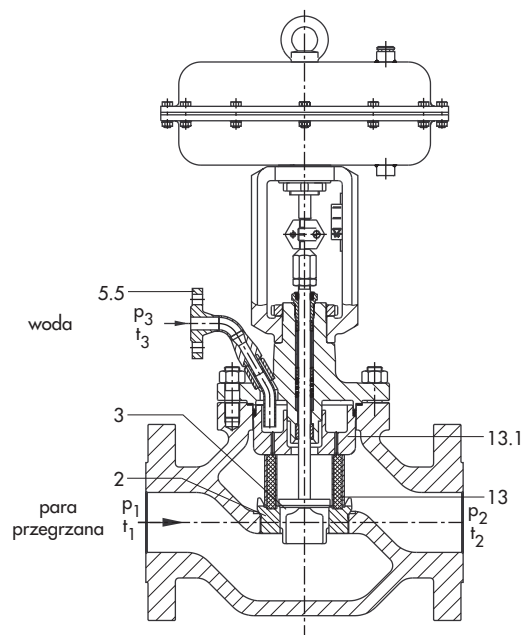
Rys. 3 · Zawór schładzający do pary typu 3281-1 z przyłączem kołnierzowym i siłownikiem typu 3271
