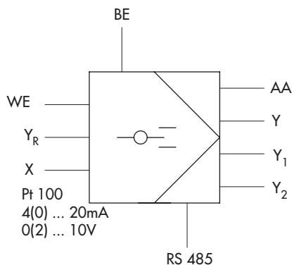
Rys. 2 · TROVIS 6497 z wyjściem sygnałów przełączających
