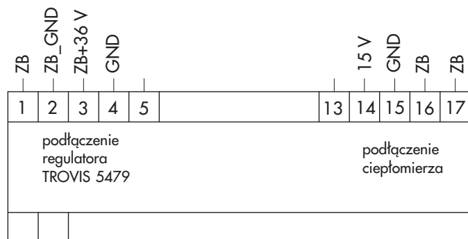
Rys. 7 · Podłączenie zacisków regulatora TROVIS 5479
