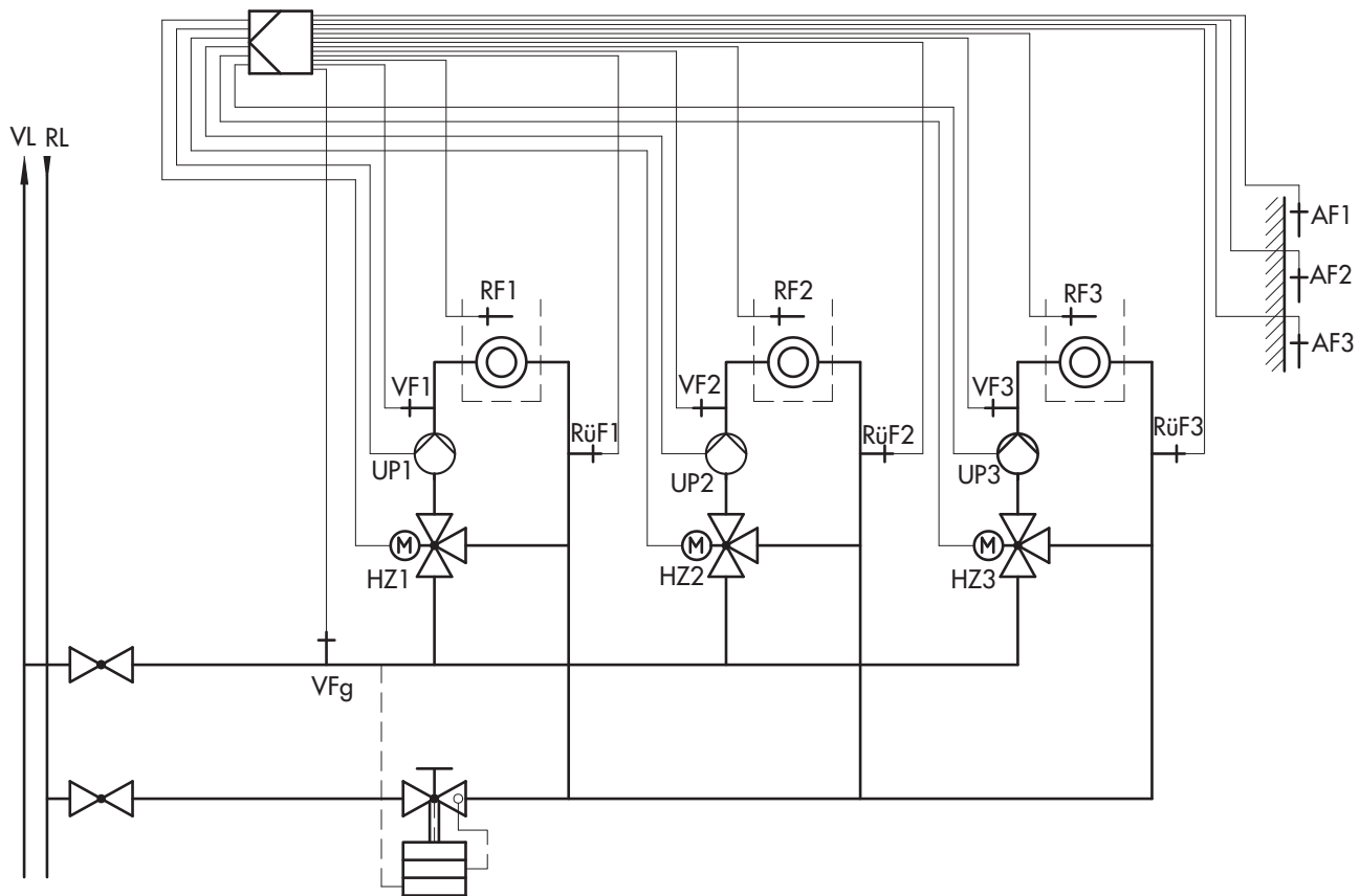
Rys. 10 · Instalacja nr 6
