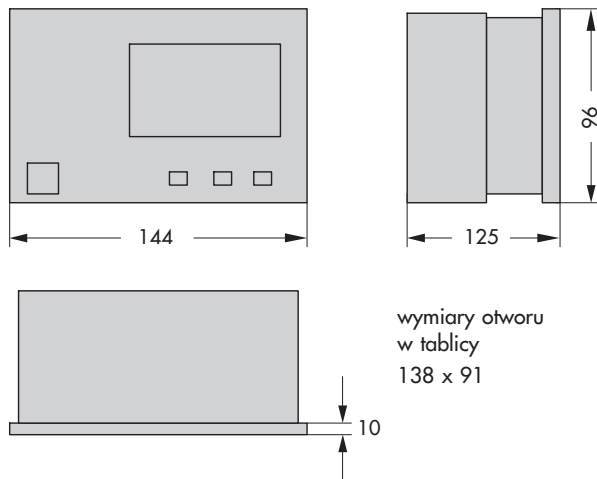
Rys. 7 · TROVIS 5479
