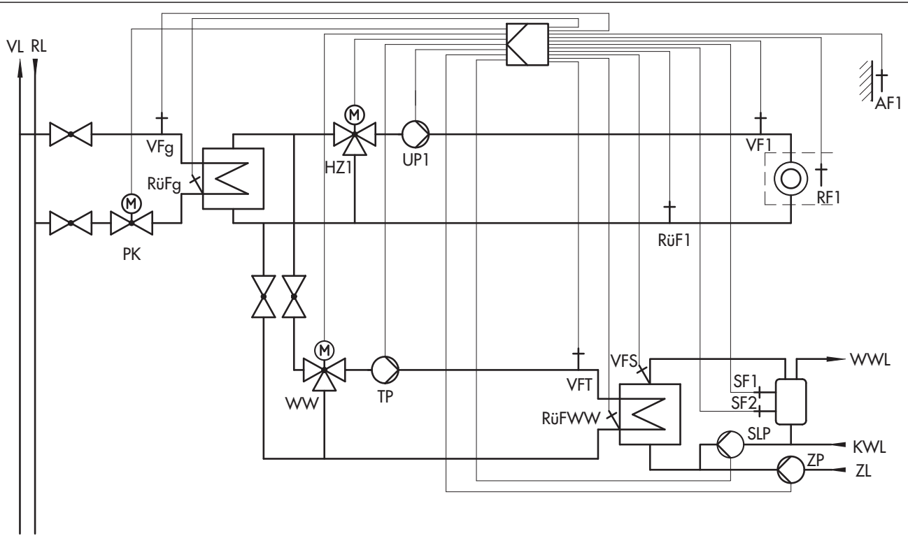
Rys. 9 · Instalacja nr 4
